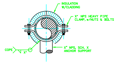
DET. 3 ANCHOR TEE CLAMP
